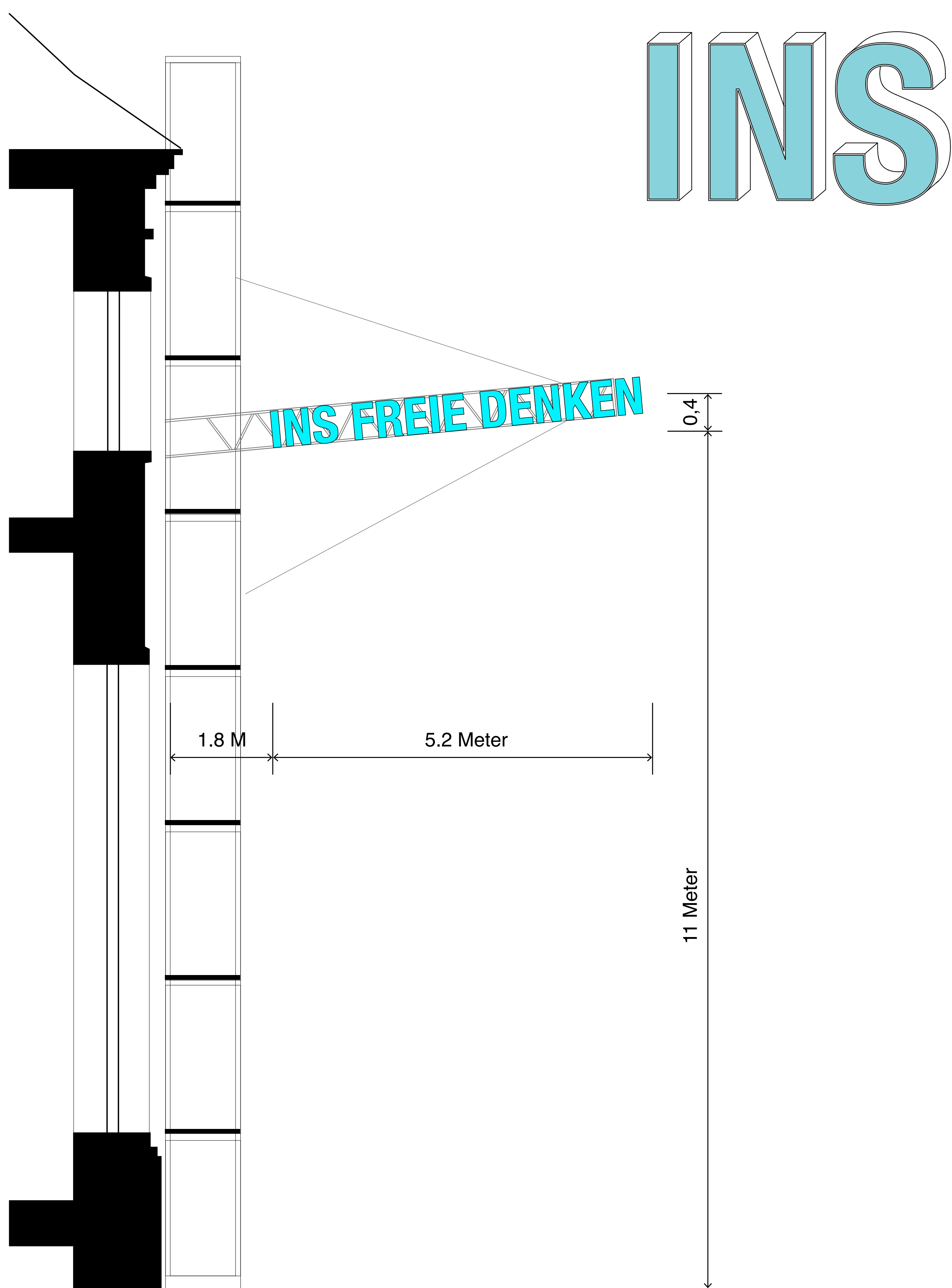
SCHNITT FASSADENGERÜST M. 1:50
